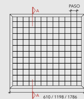
ELEVACIÓN
